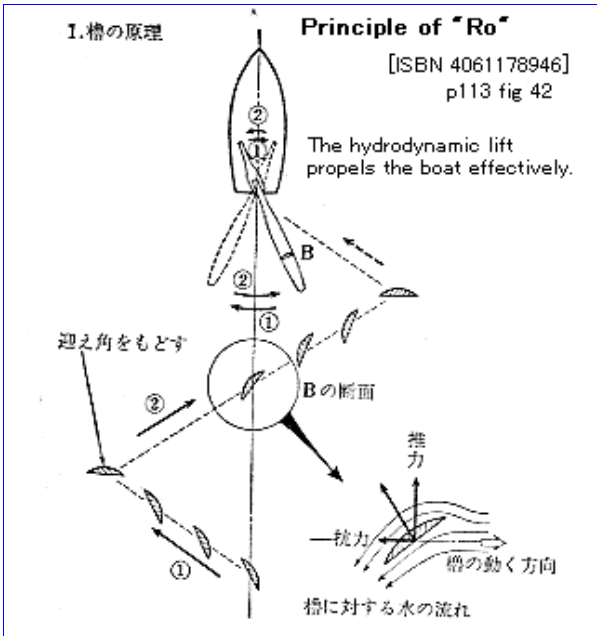
櫓の原理 (講談社ブルーバックス「船の科学」吉田文二より)
