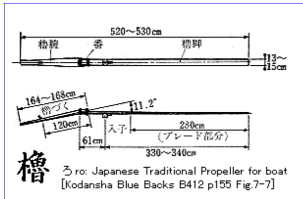
櫓の概要 (講談社ブルーバックス「生物の泳法」東昭より)
